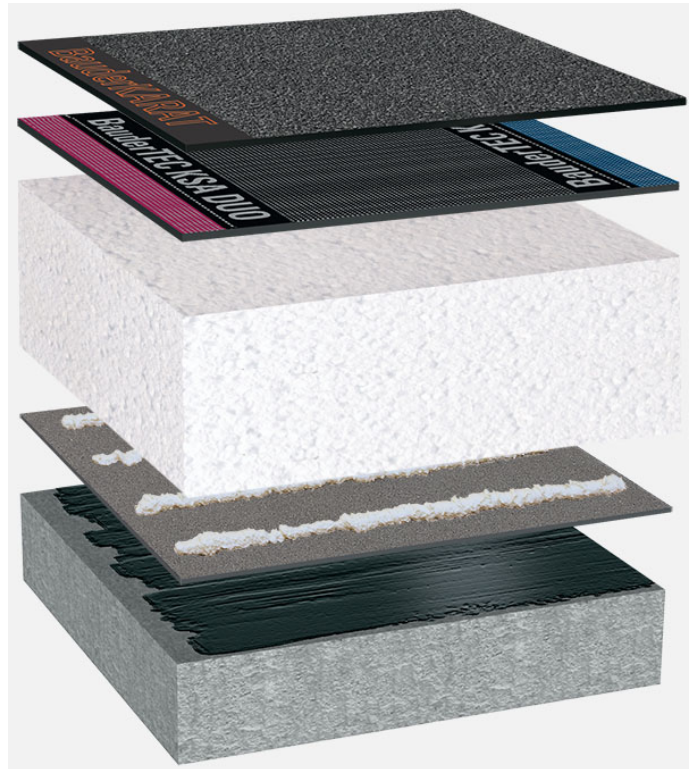
Systemaufbau: BG_EPS-P_K_01
