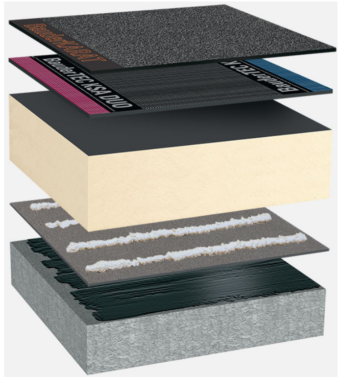
Systemaufbau: BG_PIR-FA_K_01
