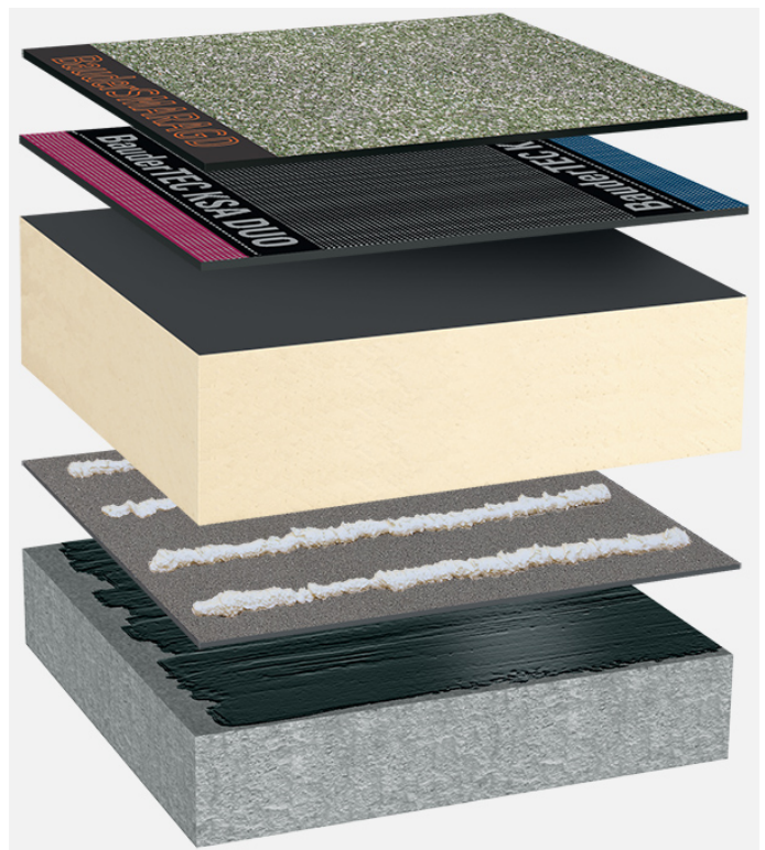
Systemaufbau: BG_PIR-FA_S_01
