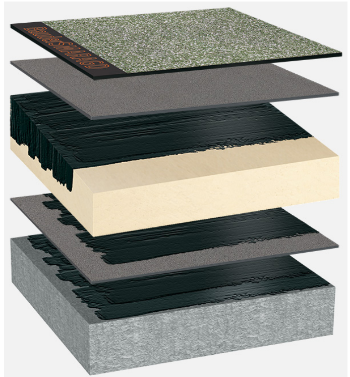
Systemaufbau: BG_PIR-KP_S_01
