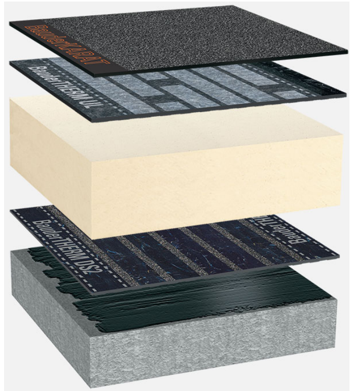
Systemaufbau: BG_PIR-MF_K_01
