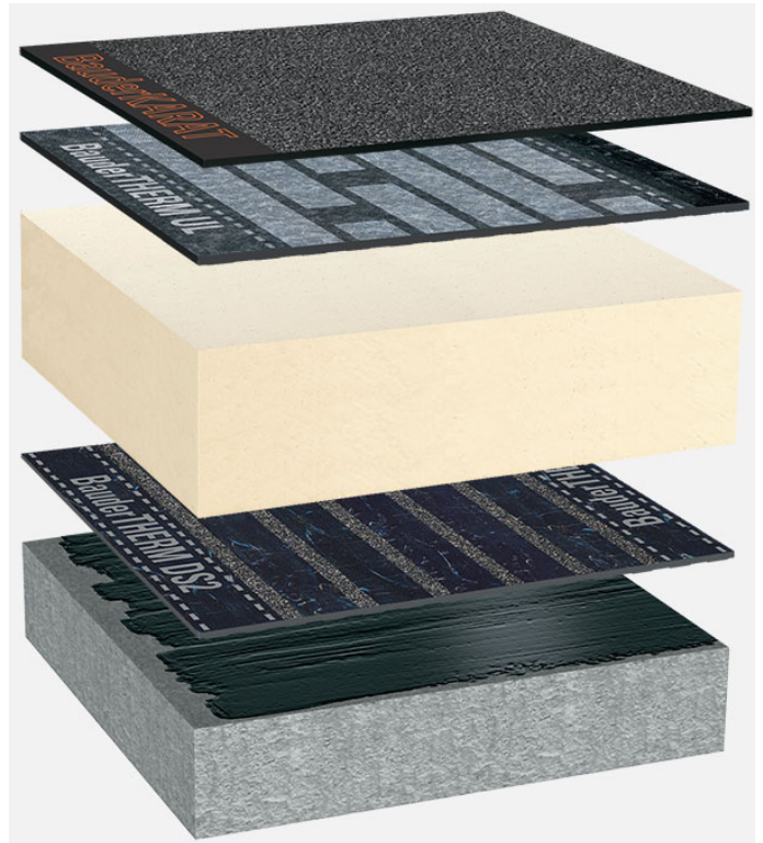
Systemaufbau: BG_PIR-MF_K_01
