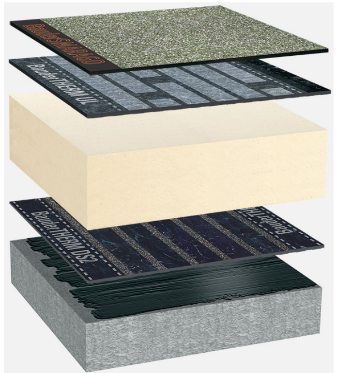
Systemaufbau: BG_PIR-MF_S_01
