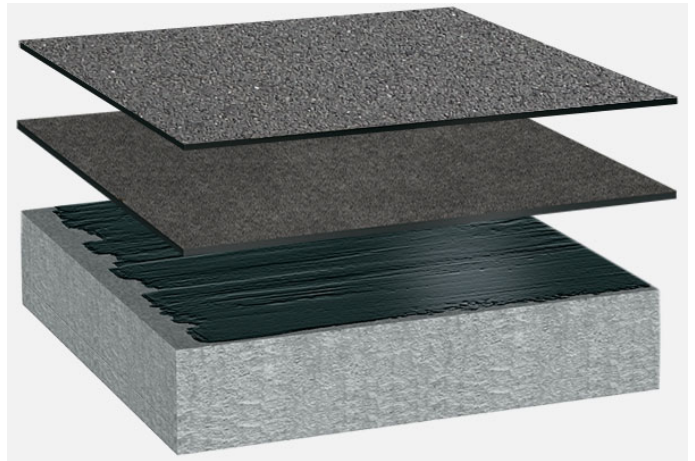
Systemaufbau: BG_B_01
