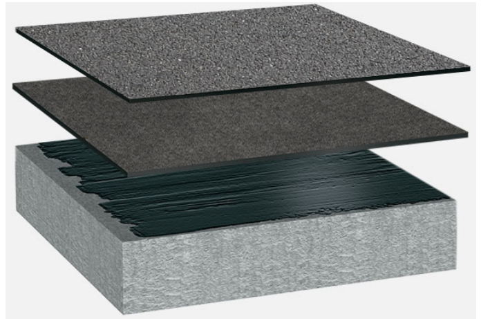
Systemaufbau: BG_B_03
