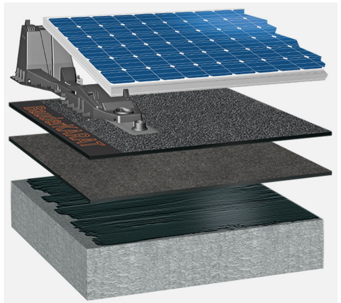
Systemaufbau: BG_K_01_PVFD
