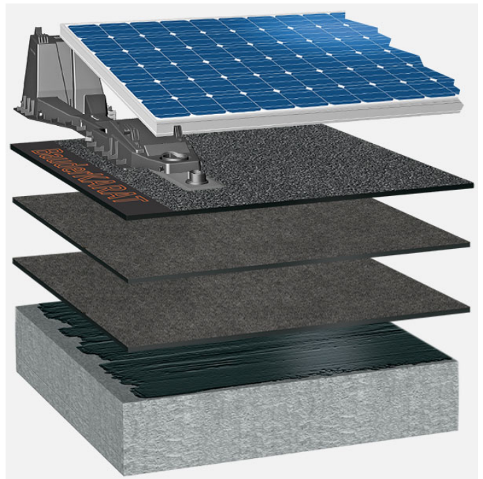
Systemaufbau: BG_K_02_PVFD
