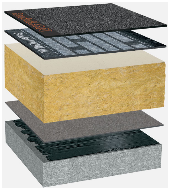
Systemaufbau: BG_MIFA-P_K_01
