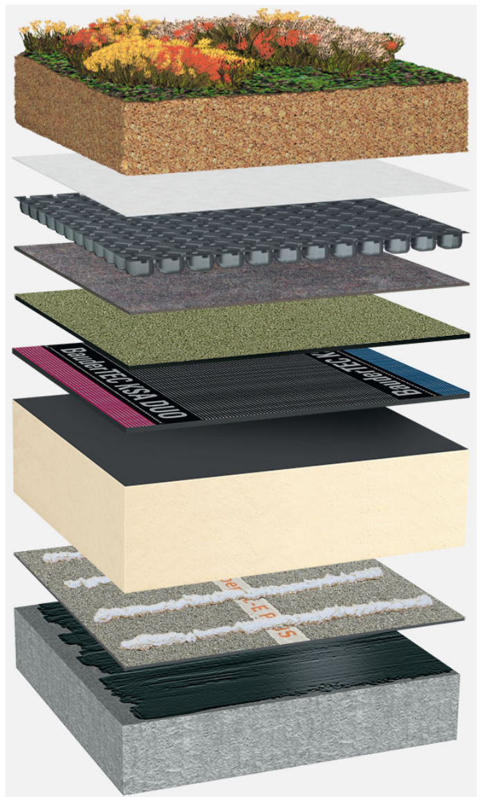
Systemaufbau: BG_PIR-FA_P_01_G125
