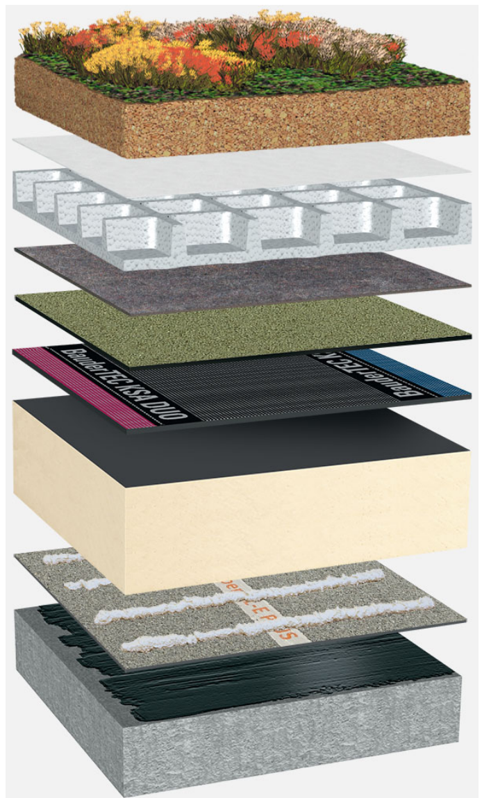
Systemaufbau: BG_PIR-FA_P_01_G75
