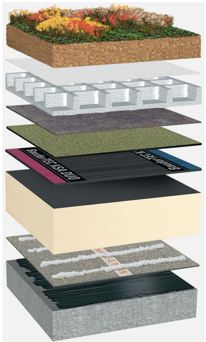
Systemaufbau: BG_PIR-FA_P_01_G75
