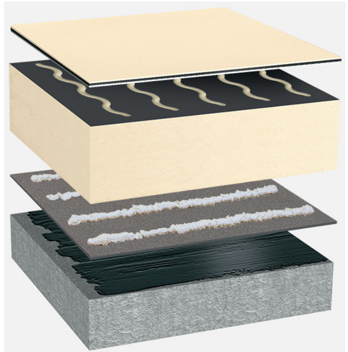
Systemaufbau: BG_PIR-FA_TV_01
