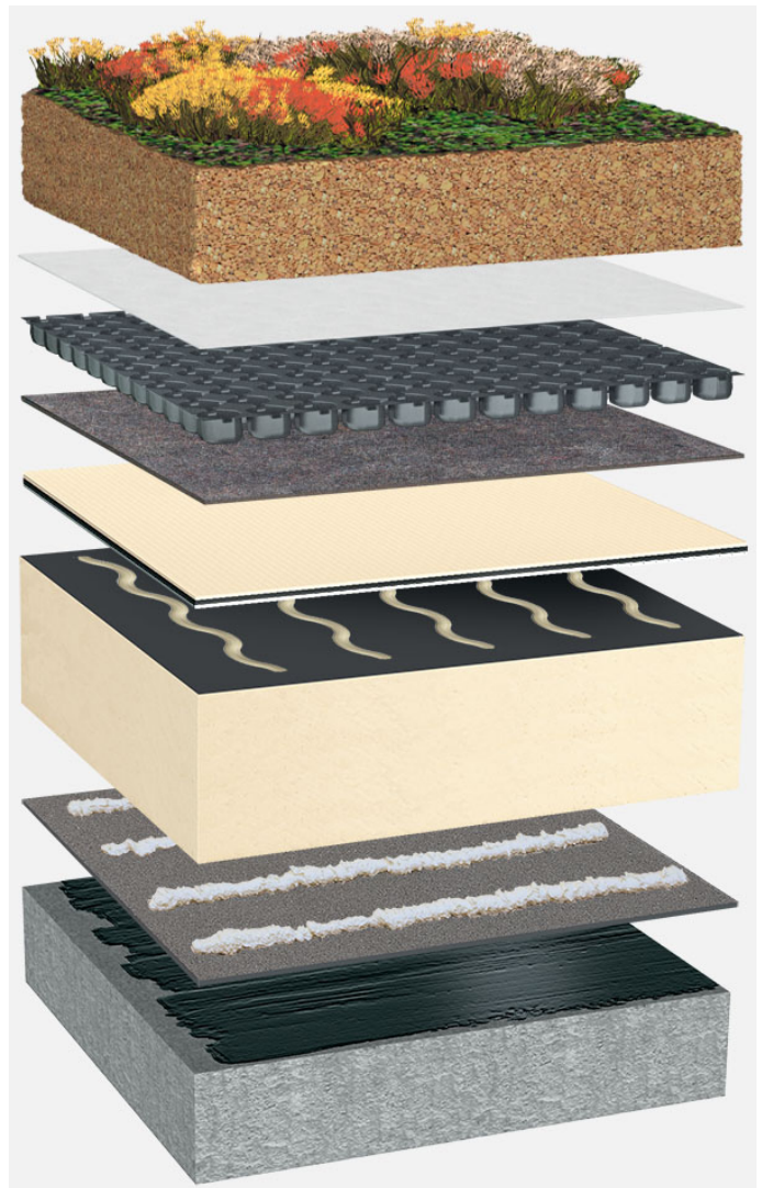
Systemaufbau: BG_PIR-FA_TV_01_G125
