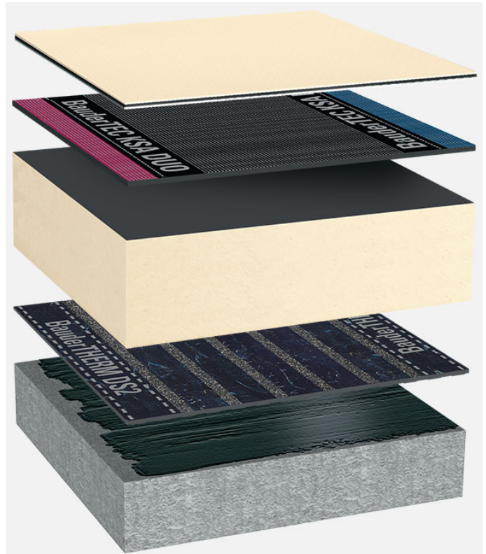
Systemaufbau: BG_PIR-FA_TV_02
