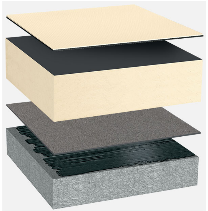
Systemaufbau: BG_PIR-FA_T_01
