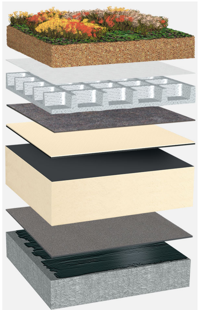
Systemaufbau: BG_PIR-FA_T_01_G75
