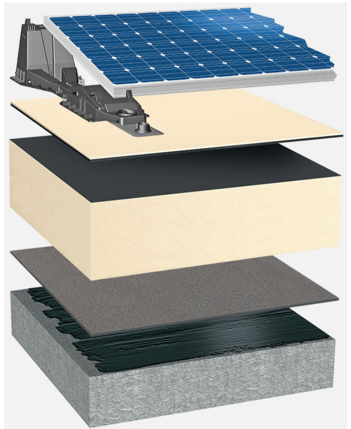
Systemaufbau: BG_PIR-FA_T_01_PVFD
