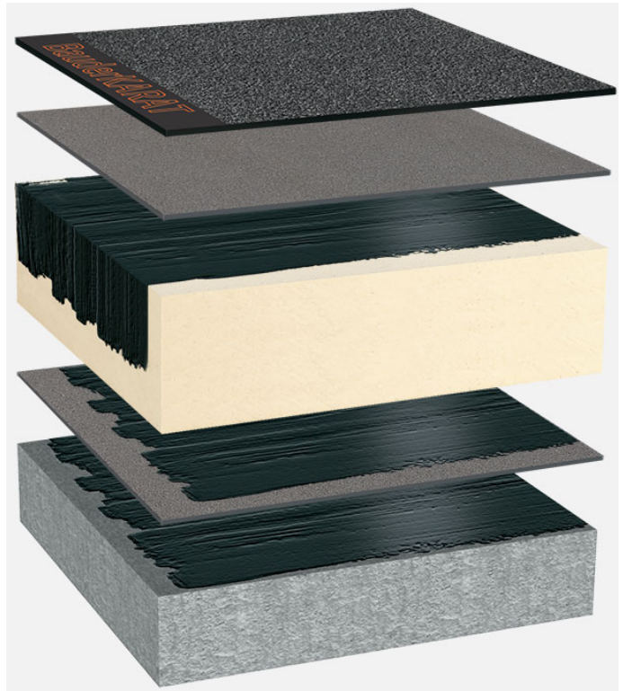
Systemaufbau: BG_PIR-KP_K_01
