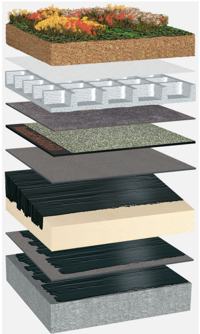
Systemaufbau: BG_PIR-KP_S_01_G75
