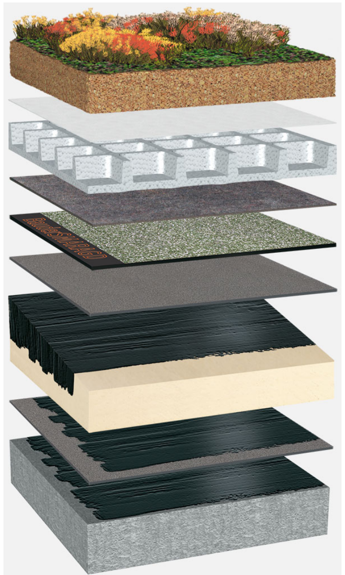
Systemaufbau: BG_PIR-KP_S_01_G75
