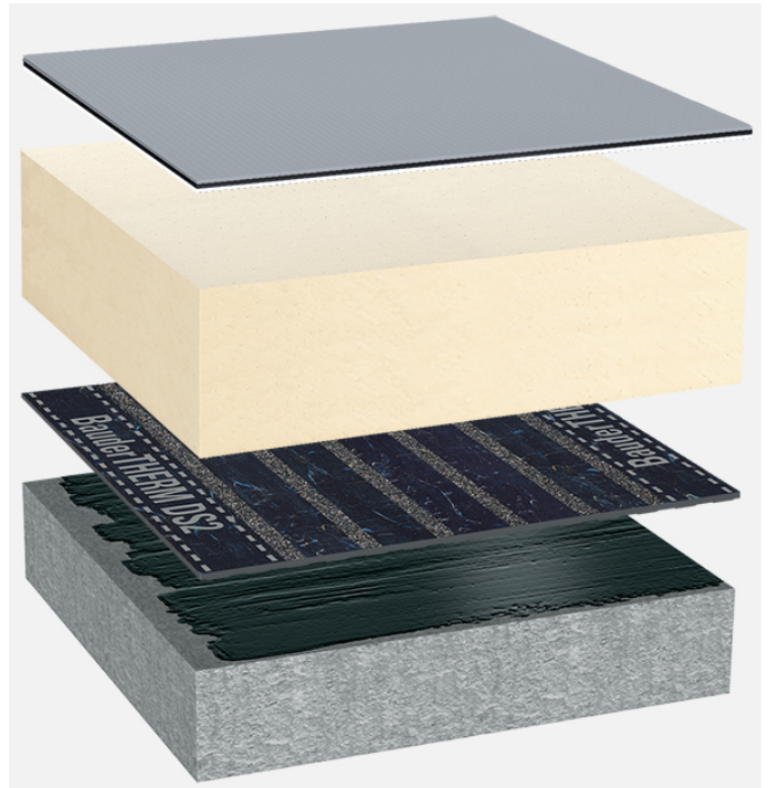
Systemaufbau: BG_PIR-MF_SK_01
