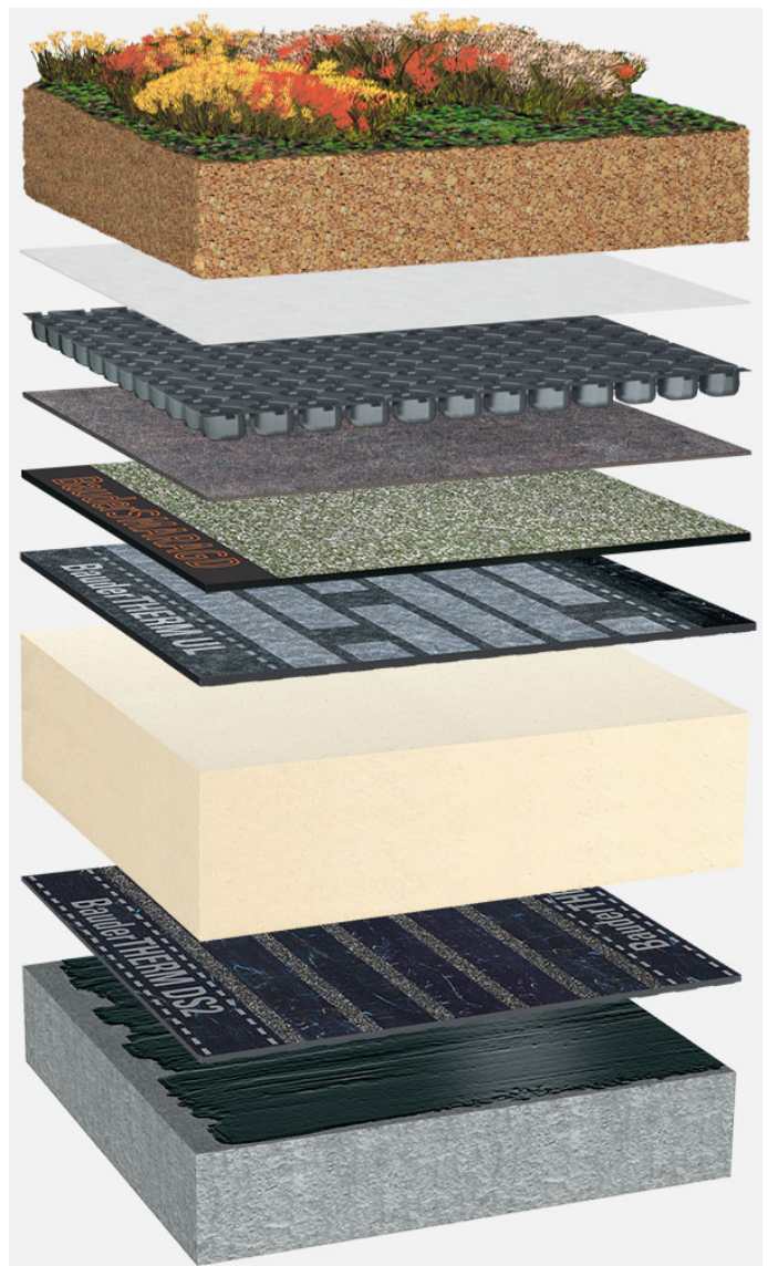
Systemaufbau: BG_PIR-MF_S_01_G125
