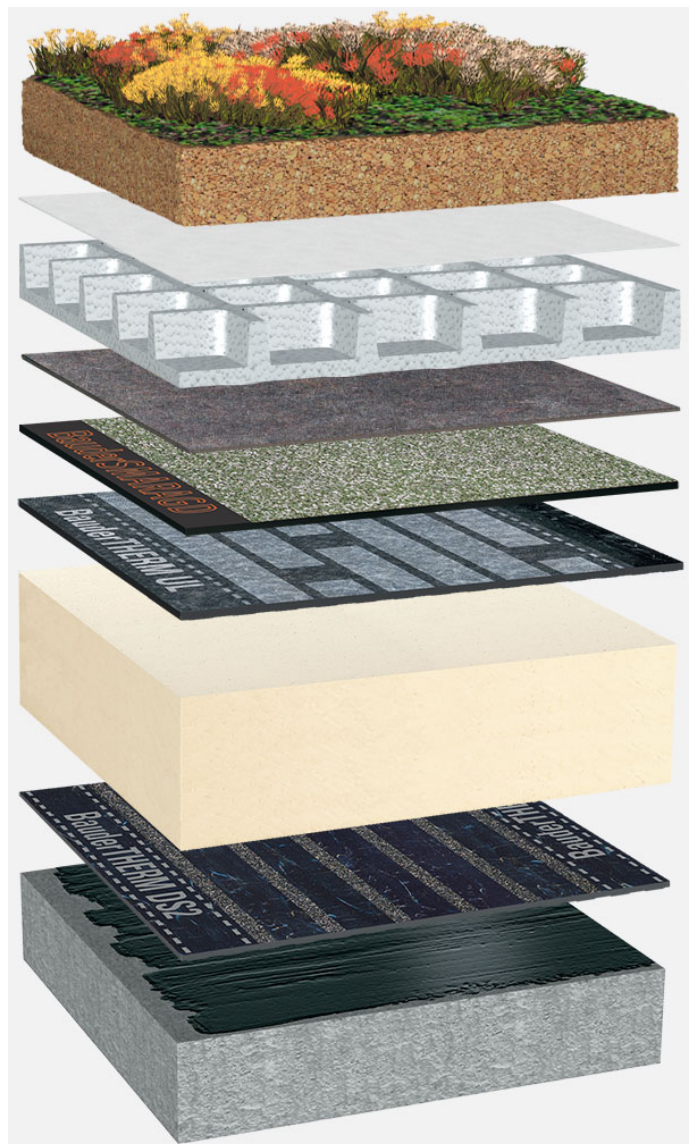
Systemaufbau: BG_PIR-MF_S_01_G75
