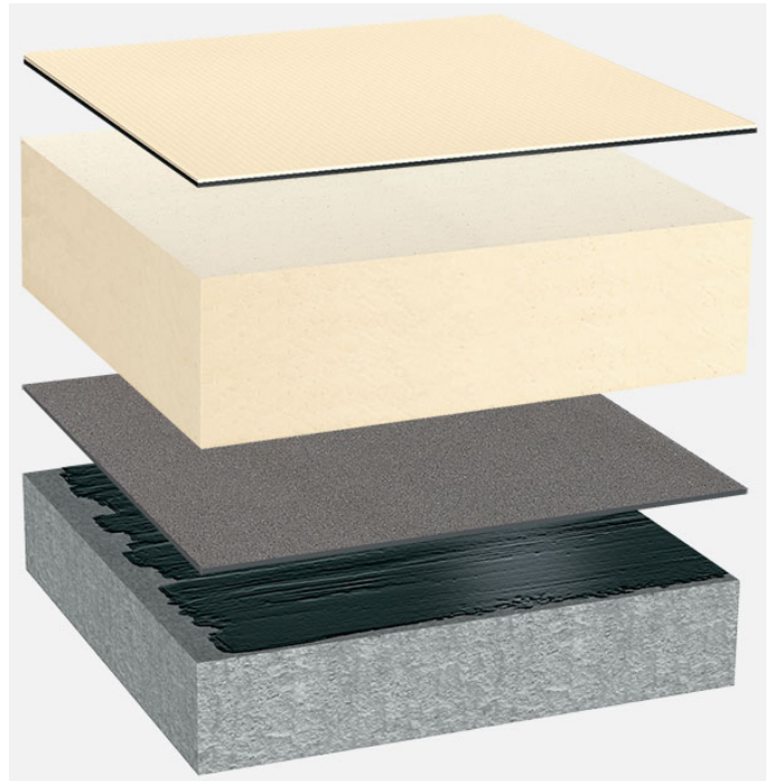
Systemaufbau: BG_PIR-MF_T_01
