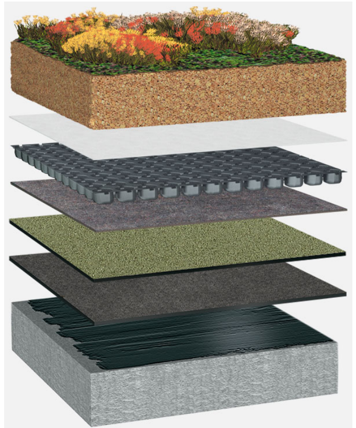
Systemaufbau: BG_P_01_G125
