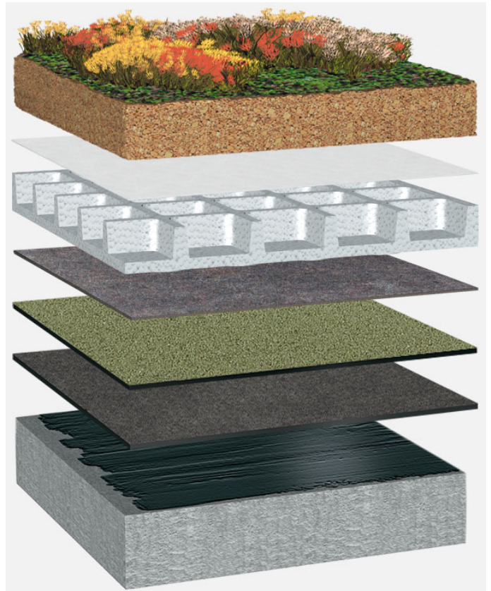
Systemaufbau: BG_P_01_G75
