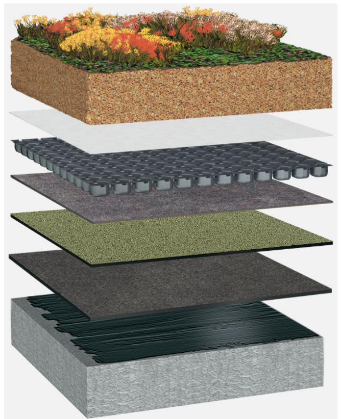
Systemaufbau: BG_P_03_G125
