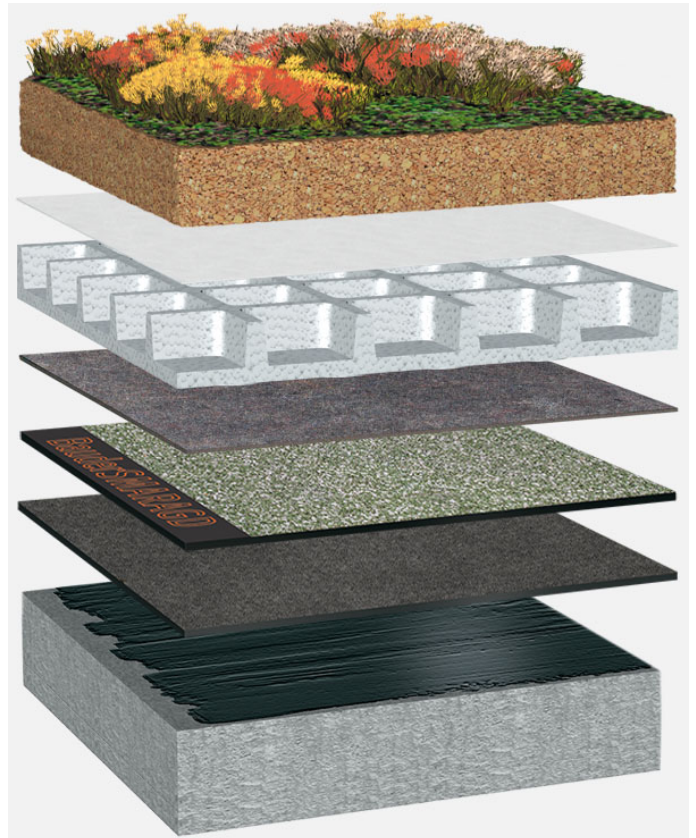
Systemaufbau: BG_S_01_G75
