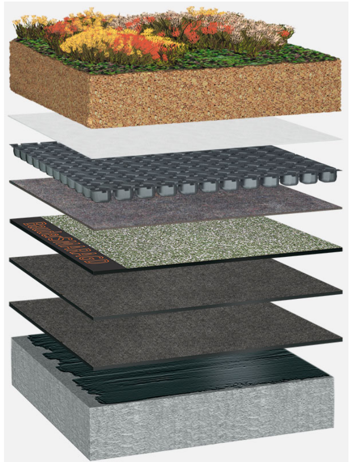
Systemaufbau: BG_S_02_G125
