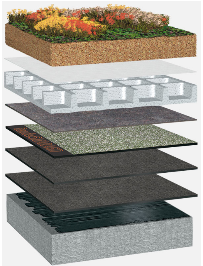
Systemaufbau: BG_S_02_G75
