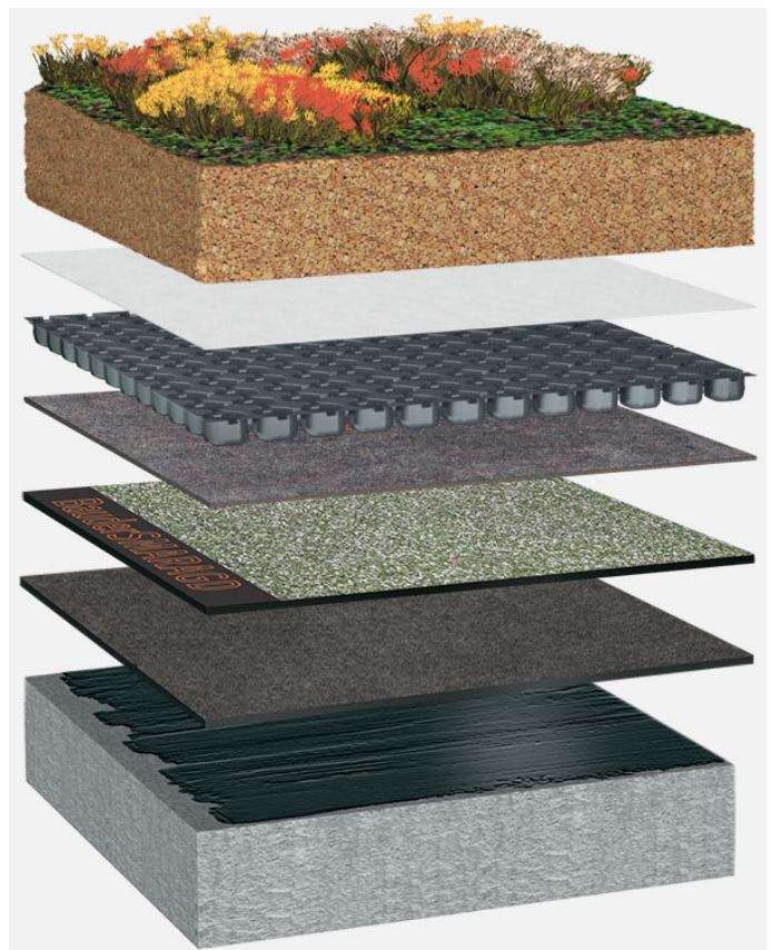
Systemaufbau: BG_S_03_G125
