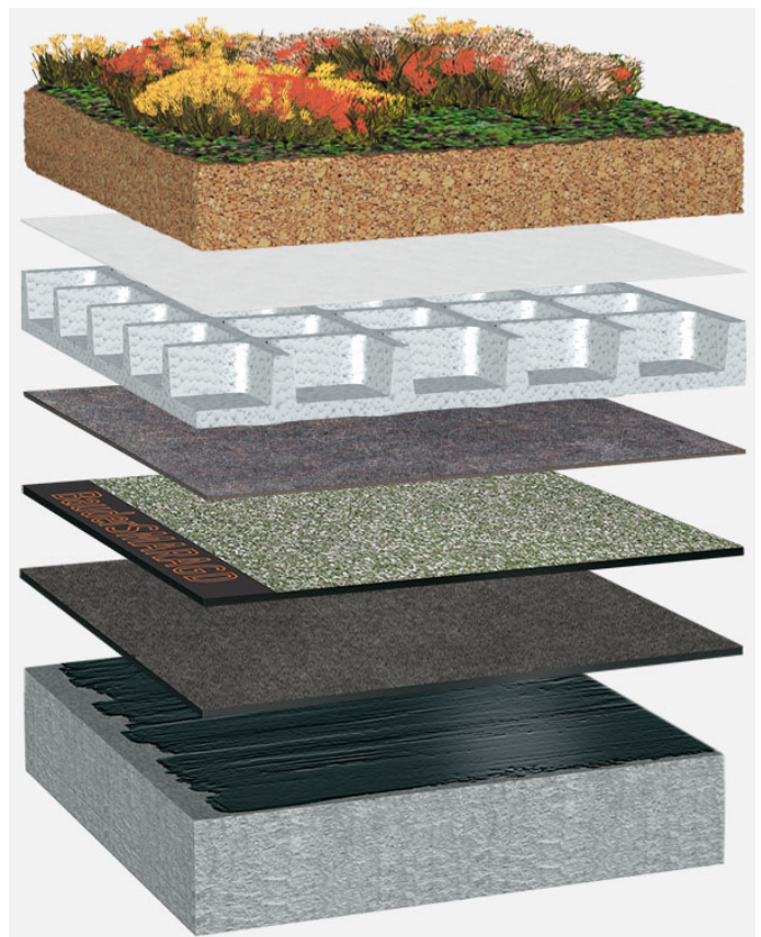
Systemaufbau: BG_S_03_G75
