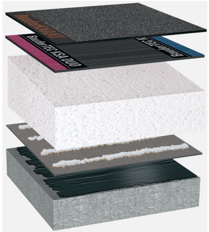
Systemaufbau: BP_EPS-G_K_01
