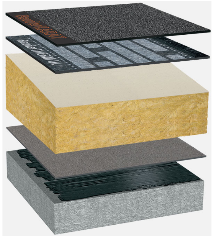
Systemaufbau: BP_MIFA-G_K_01
