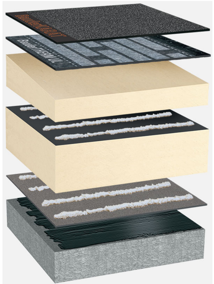
Systemaufbau: BP_PIR-FA_PIR-TG_K_01
