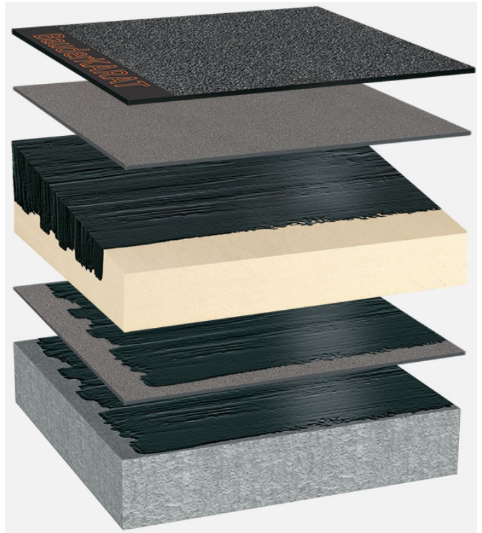
Systemaufbau: BP_PIR-KG_K_01
