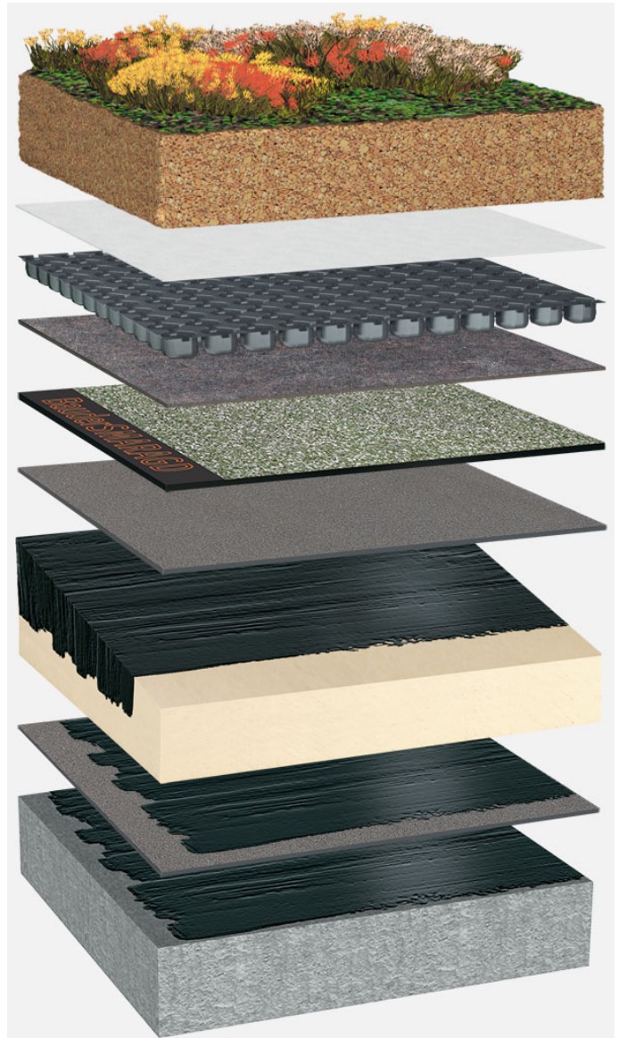
Systemaufbau: BP_PIR-KG_S_01_G125
