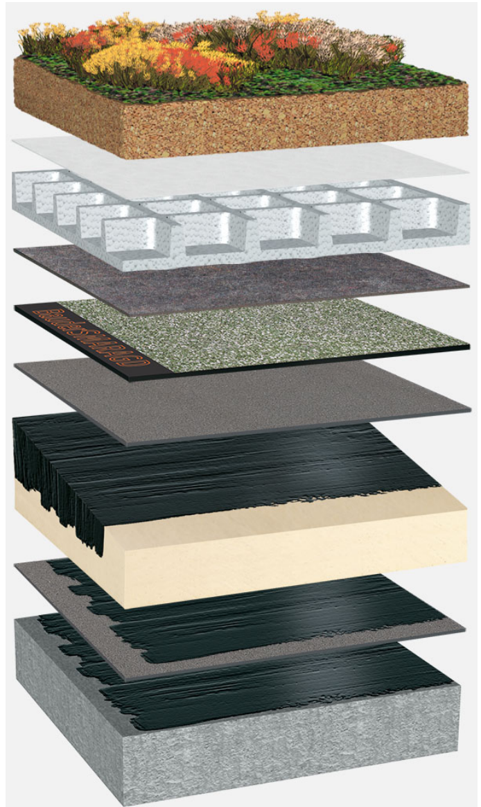
Systemaufbau: BP_PIR-KG_S_01_G75
