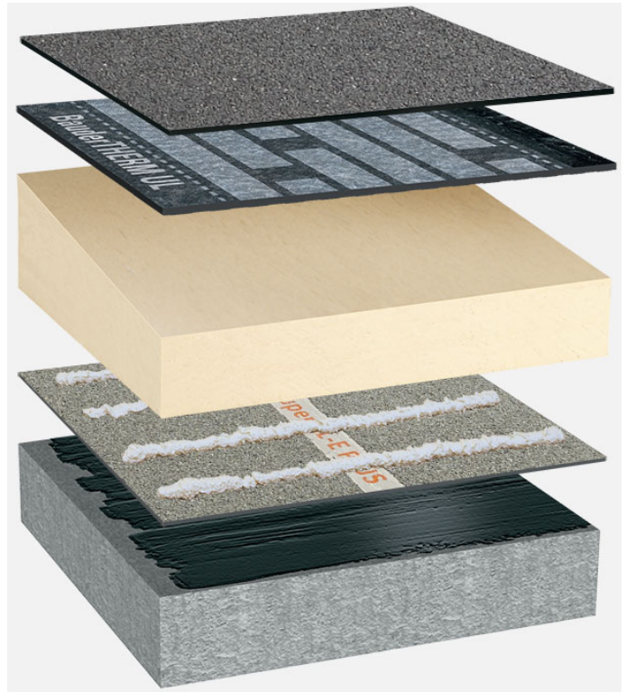
Systemaufbau: BP_PIR-TG_B_01
