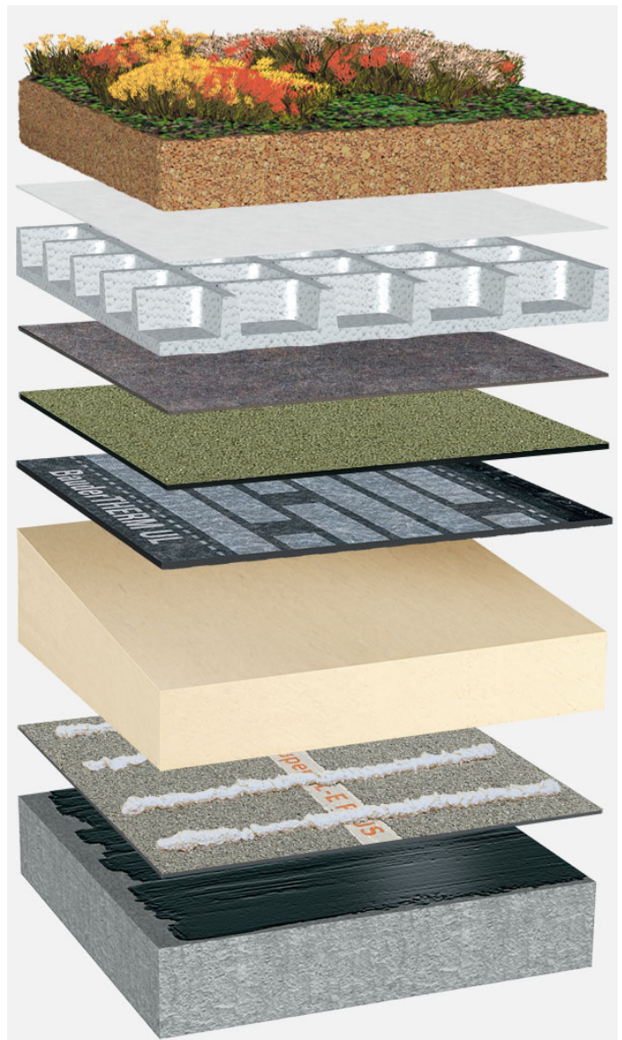
Systemaufbau: BP_PIR-TG_P_01_G75
