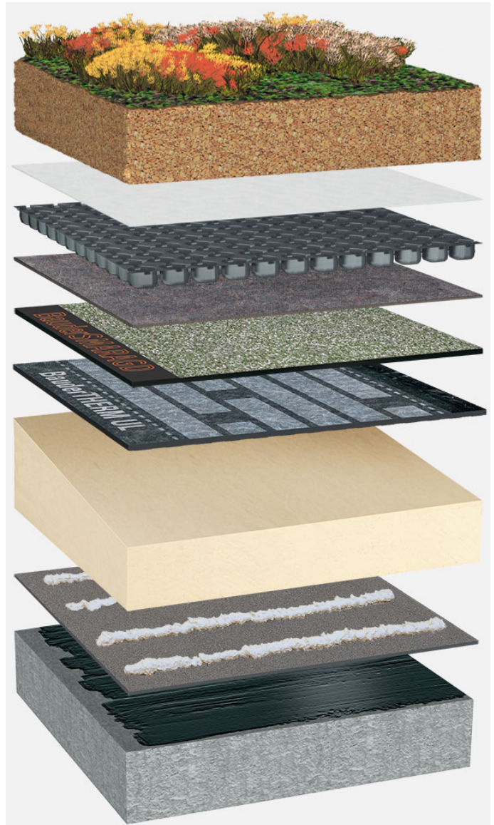
Systemaufbau: BP_PIR-TG_S_01_G125
