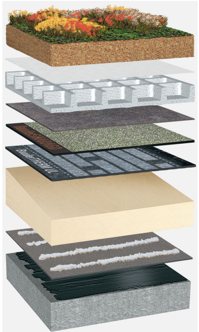
Systemaufbau: BP_PIR-TG_S_01_G75
